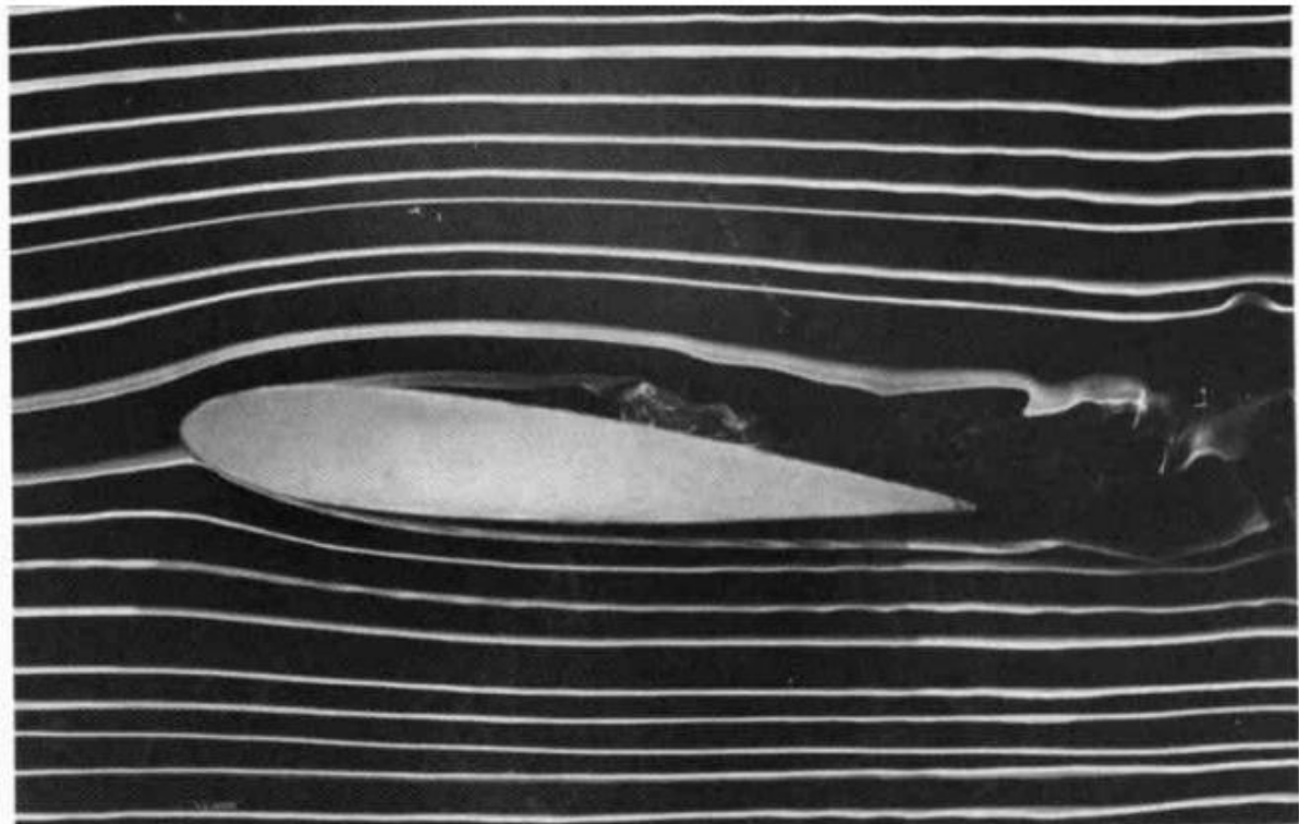
LIGNES DE CHAMP AUTOUR D'UN PROFIL D'AILE
