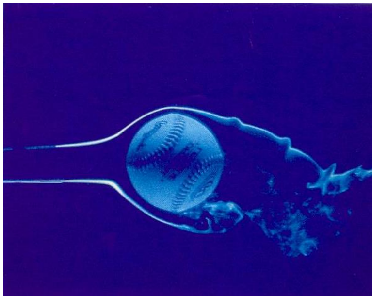
Ecoulement d'eau autour d'une balle de base ball en rotation
