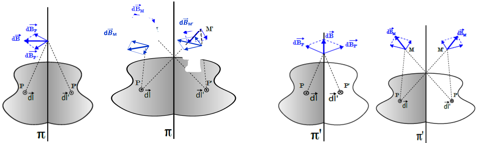
Champ magnétique et plan de symétrie...
