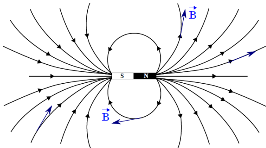
Lignes de champ d'un aimant droit
