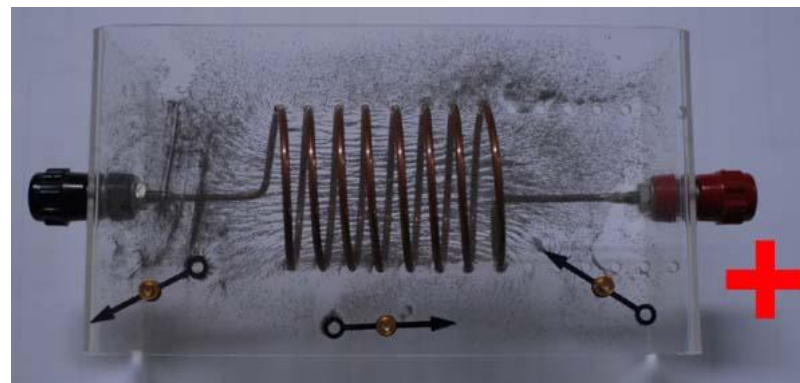
Lignes de champ d'un ensemble de spires coaxiales
