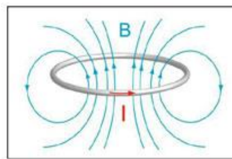
Spire de courant
