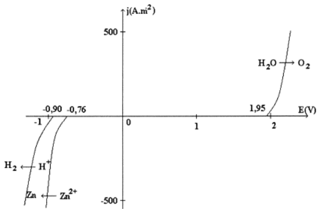
Figure 6 : courbes intensité-potentiel pour l'eau et les ions zinc
