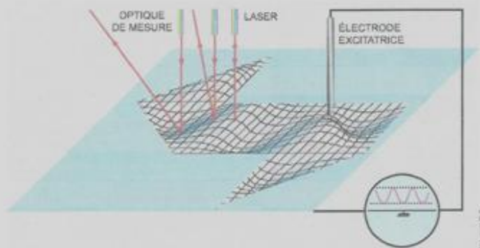
4. DISPOSITIFS D'EXCITATION ET DE DÉTECTION des vibrations d'une membrane. L'excitation est obtenue au moyen d'une électrode. La partie continue de la tension attire les charges de la membrane, qui s'accumulent sous l'électrode. La composante alternative de la tension exerce alors une force électrostatique sinusoïdale. La détection utilise la réflexion d'un faisceau laser sur la surface de la membrane.
